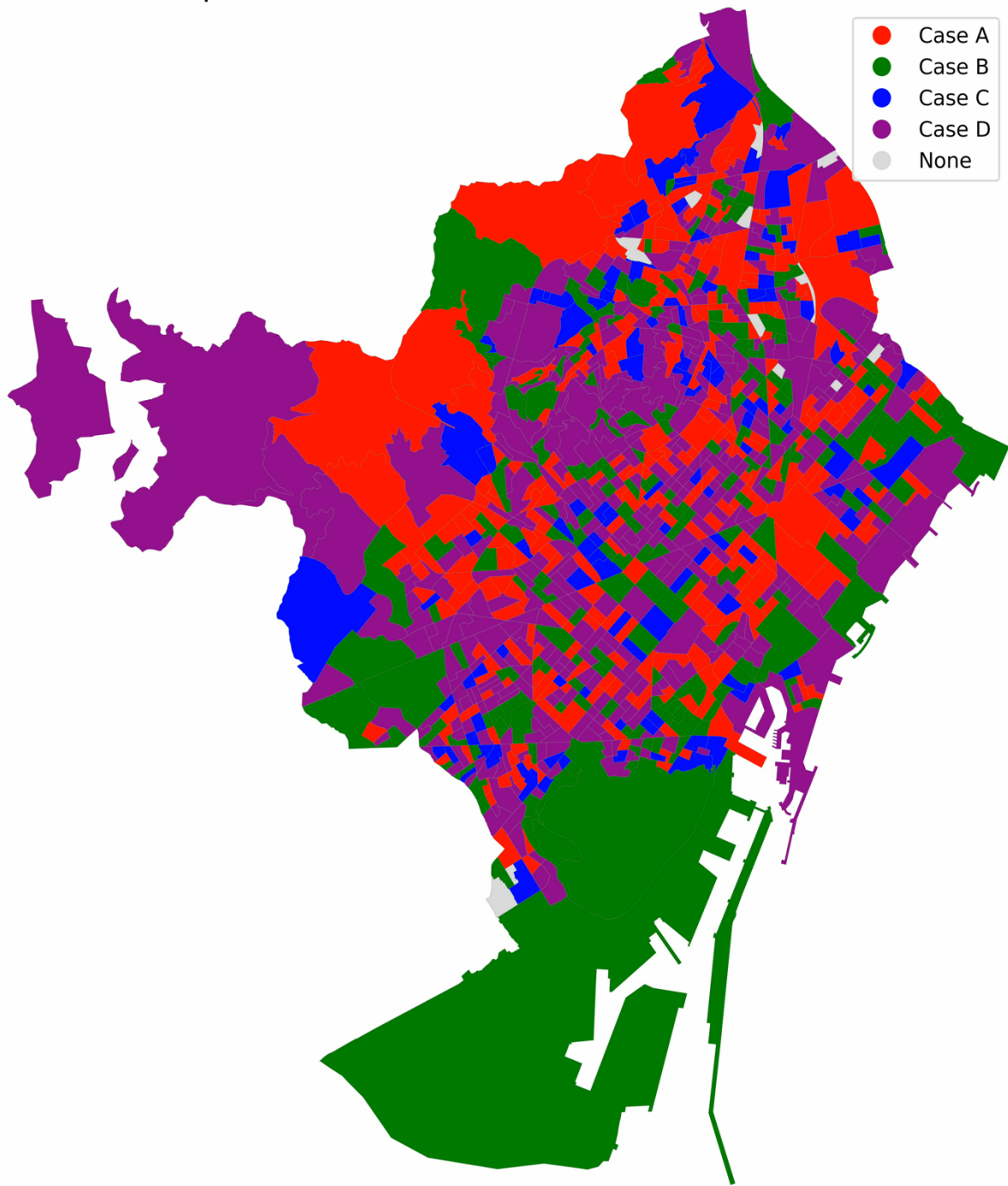
Gráfico 12: Mapa de calor de gentrificación en la Ciudad de Barcelona entre los años 2012 y 2022.
